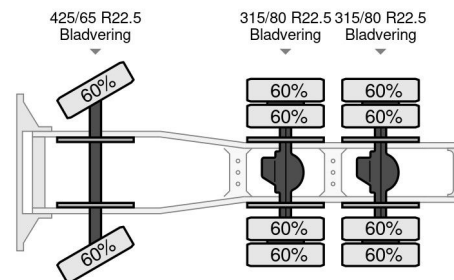
Mercedes-Benz 2644 - V8 6x4
