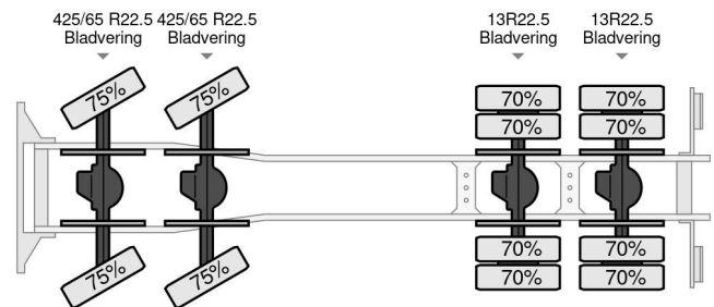
Mercedes-Benz Actros 4140 AK - 8x8
