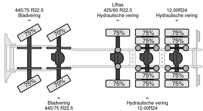
Ginaf X 5450 S - 10x8 MANUAL GEAR
