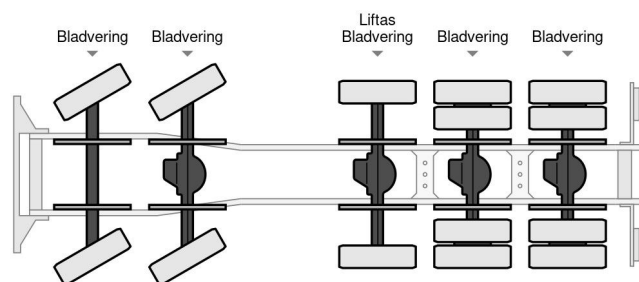
Mercedes-Benz Actros 5044 AK - 10x8
