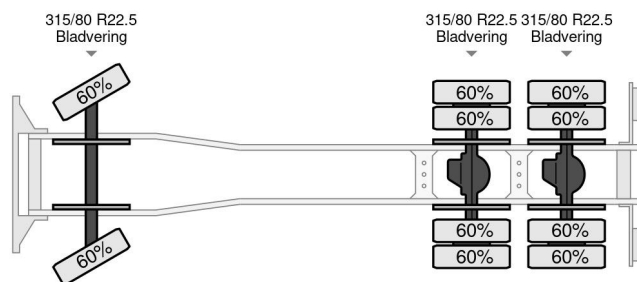
Mercedes-Benz 3335 Actros - 6x4 - Haak / Hooksystem
