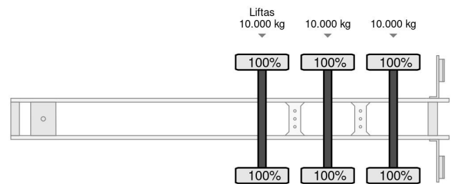
ATM 15-30 met oprolzeil - 2 Assen gestuurd - Liftas
